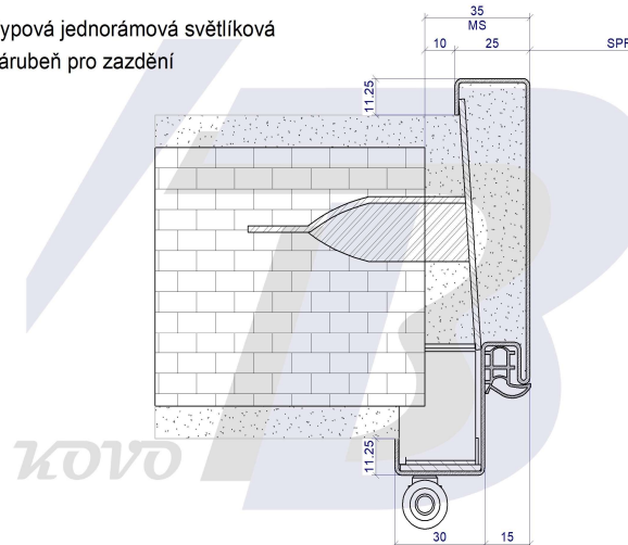
Typová jednorámová univerzální zárubeň pro montáž svarem
