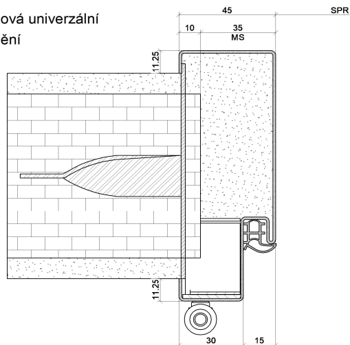
Typová jednorámová světlíková zárubeň pro zazdění
