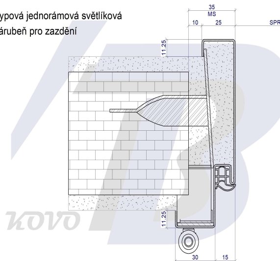
Typová jednorámová univerzální zárubeň pro montáž svarem
