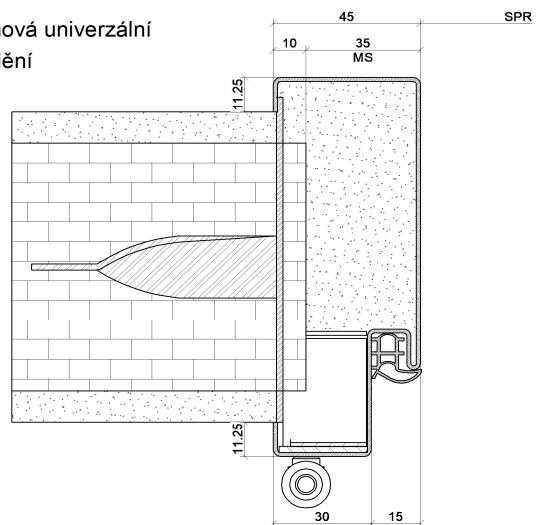
Typová jednorámová světliková zárubeň pro zazdění
