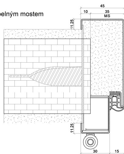
Typová světlíková zárubeň s přerušeným tepelným mostem pro zazdění
