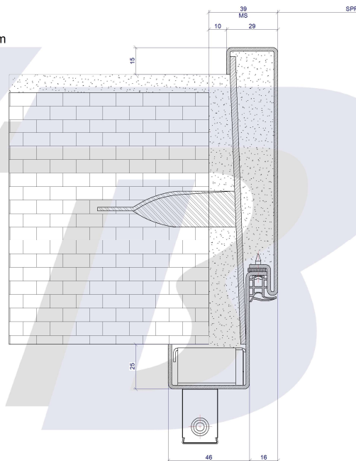
Systémová zárubeň s přerušeným tepelným mostem pro montáž svarem
