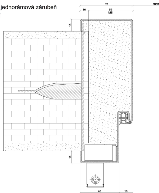
Systémová jednorámová světlíková zárubeň pro zazdění
