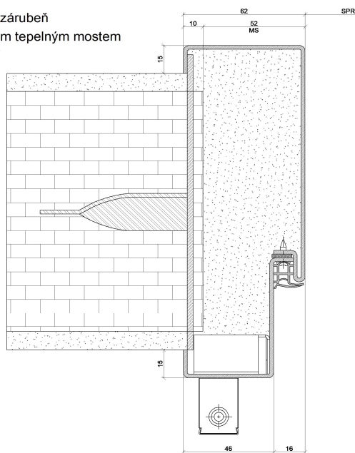
Systémová světlíková zárubeň s přerušeným tepelným mostem pro zazdění
