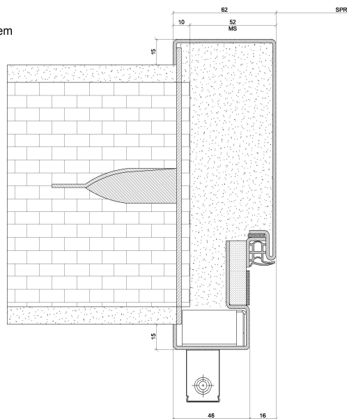
Systémová světlíková zárubeň s přerušeným tepelným mostem pro zazdění
