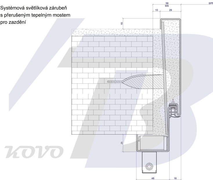
Systémová zárubeň s přerušeným tepelným mostem pro montáž svarem
