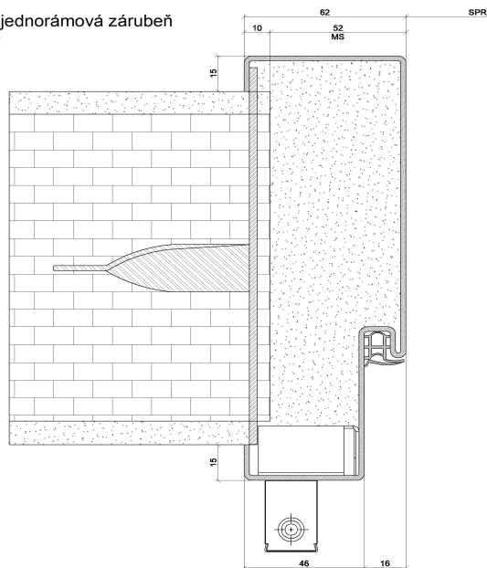
Systémová jednorámová světlíková zárubeň pro zazdění
