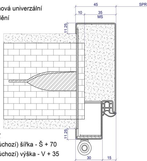
Typová jednorámová světlíková zárubeň pro zazdění
