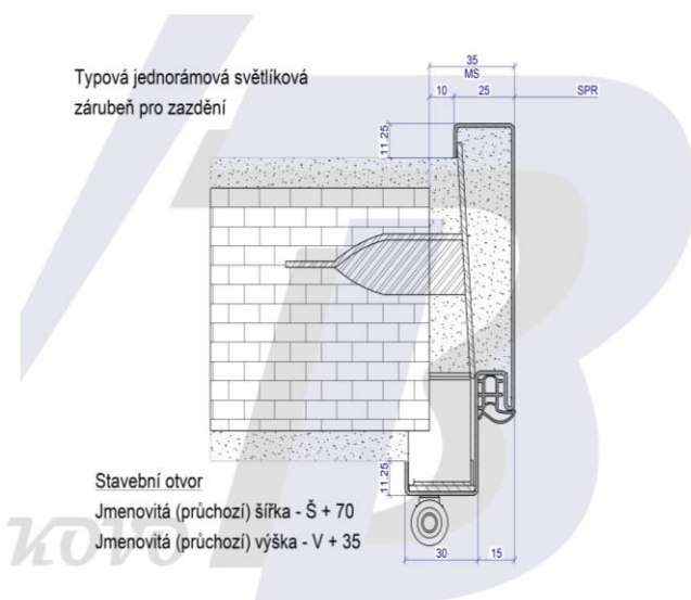
Typová jednorámová univerzální zárubeň pro montáž svarem
